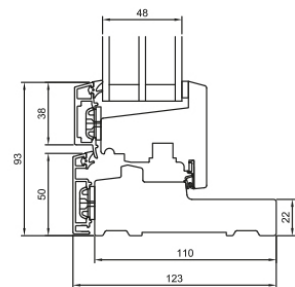
L25 Fußschwelle Holz
