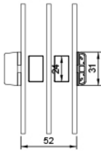
31 mm Sprosse
