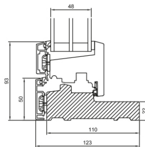
L25 Fußschwelle Hartholz
