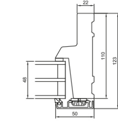
L6 Seitlicher Blendrahmen Unterlicht
