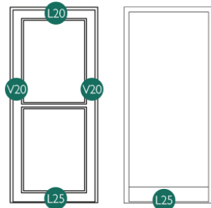
L20 Oberer Blendrahmen/Flügel
