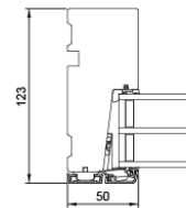
V6 Seitlicher Blendrahmen Oberlicht
