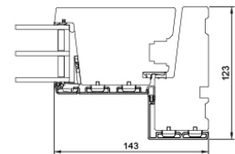
V20 Seitlicher Blendrahmen/Schließseite/Flügel
