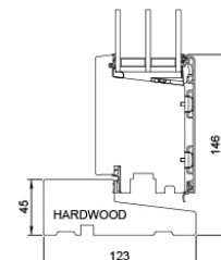
L25 Fußschwelle Holz
