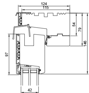
L32 Oberer Blendrahmen mit Flügel
