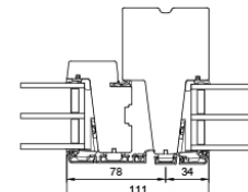
V11 Seitlicher Blendrahmen/ Seitenteil
