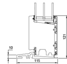
L25 Fußschwelle Standard
