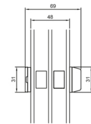
31 mm Sprosse
