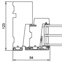
V1 Seitlicher Blendrahmen/ Flügel
