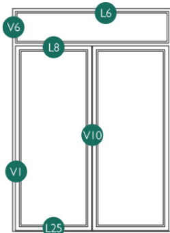
L6 Oberer Blendrahmen Oberlicht
