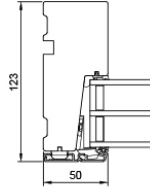
V6 Seitlicher Blendrahmen
