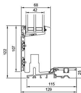
L34 Fußschwelle beweglicher Teil
