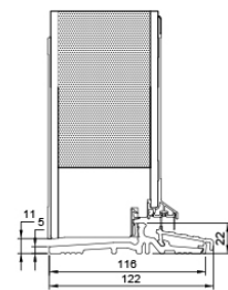
L25 Fußschwelle Standard bei Plattentüren
