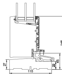
L25 Fußschwelle Holz – auf Wunsch, nur bei Rahmentüren
