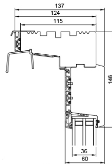
L31 Oberer Blendrahmen fester Teil
