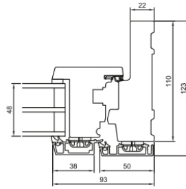
V1 Seitlicher Blendrahmen/Flügel
