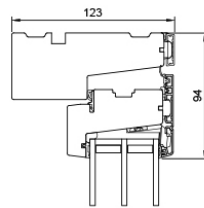
L1 Oberer Blendrahmen/ Flügel
