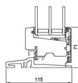
L25 Fußschwelle Tür Standard
