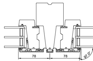
V2 A: Mittlerer Anschlag mit Pfosten B: Mittlerer Anschlag Topschwingfenster
