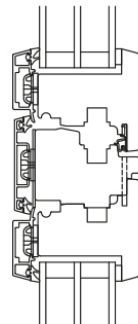
V22 Stulpausführung
