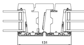
V10 Mittlerer Anschlag Stulp
