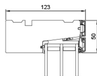
L6 Oberer Blendrahmen Oberlicht
