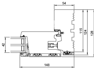
V32 Seitlicher Blendrahmen/Flügel
