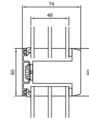
60 mm Sprosse
