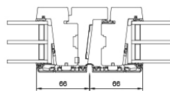
V10 Mittlerer Anschlag Stulp
