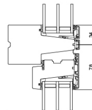
L8 Kämpfer, Flügel/ Oberlicht
