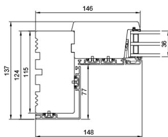
V30 Seitlicher Blendrahmen fester Teil
