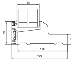
L3 Fußschwelle Unterlicht
