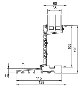
L33 Fußschwelle fester Teil
