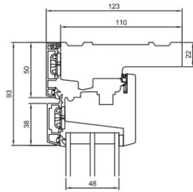
L1 Oberer Blendrahmen/Flügel
