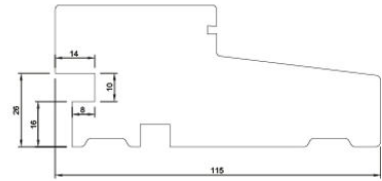
L12 Fensterbankfalz
