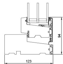
L9 Unterer Blendrahmen/ Flügel
