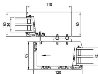
V31 Mittelposten/Flügel
