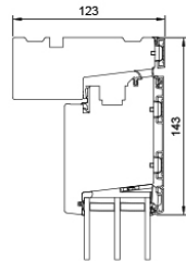
L20 Oberer Blendrahmen/ Flügel
