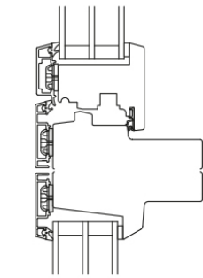
L9 Kämpferprofil Flügel/Festelement
