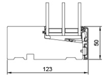
L3 Unterer Blendrahmen
