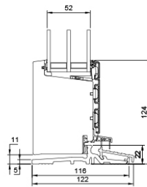
L25 Fußschwelle Standard
