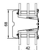
Sprosse
