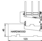
L25 Fußschwelle Tür Holz
