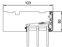
L6 Oberer Blendrahmen
