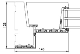
V20 Seitlicher Blendrahmen, Scharnierseite/Flügel
