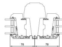
V2 A: Mittlerer Anschlag mit Posten B: Mittlerer Anschlag Topschwingfenster
