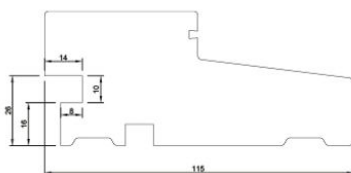
L12 Fensterbankfalz
