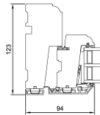
V1 Seitlicher Blendrahmen/ Flügel
