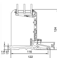
L25 Fußschwelle
