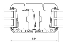
V10 Mittlerer Anschlag Stulp
