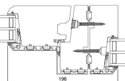
V26 Seitlicher Blendrahmen, Schließseite/Seitenteil
