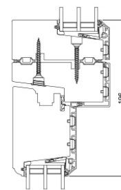
L27 Kämpfer/Flügel
