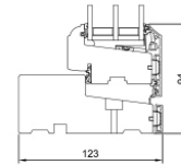
L9 Unterer Blendrahmen/ Flügel
