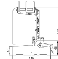
L25 Fußschwelle Holz
