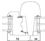
V4 Fester Blendrahmen/Flügel
