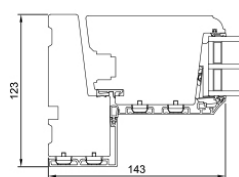
V20 Seitlicher Blendrahmen, Scharnierseite/Flügel
