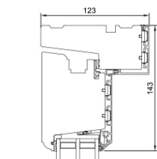
L20 Oberer Blendrahmen/ Flügel
