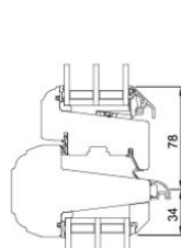
L11 Fester Blendrahmen/Flügel
