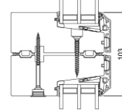
L7 Kämpferprofil
