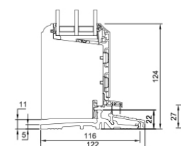
L25 Fußschwelle Standard
