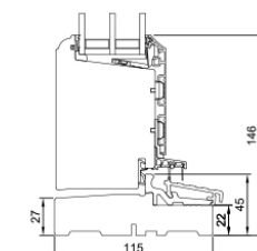
L25 Fußschwelle Holz
