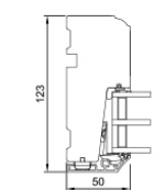
V6 Seitlicher Blendrahmen
