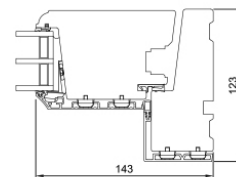
V20 Seitlicher Blendrahmen, Schließseite/Flügel
